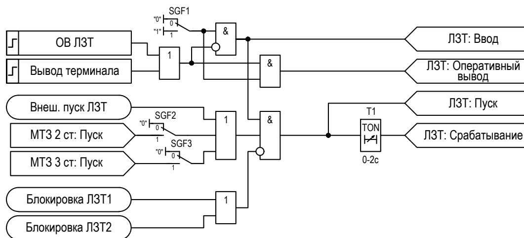
Рисунок 2.6 – Функциональная схема логики ЛЗТ
