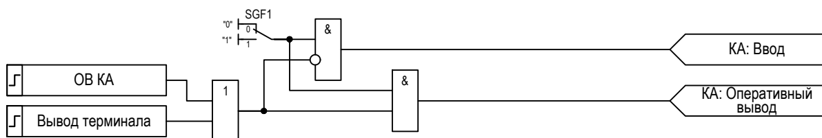
Рисунок 2.26 – Логика управления режимами функционального блока «КА»
