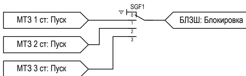
Рисунок 2.4 – Функциональная схема логики БЛЗШ
