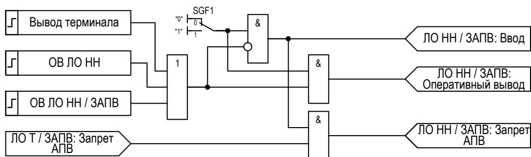
Рисунок 2.18 – Функциональная схема логики запрета АПВ
