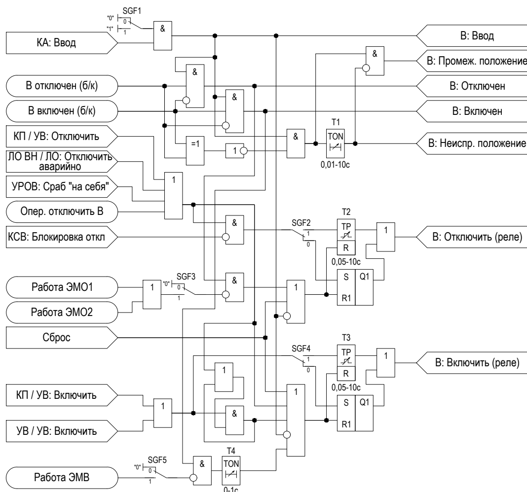
Рисунок 2.27 – Функциональная схема логики выключателя
