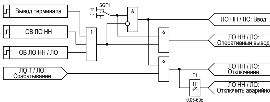
Рисунок 2.17 – Функциональная схема логики отключения выключателя
