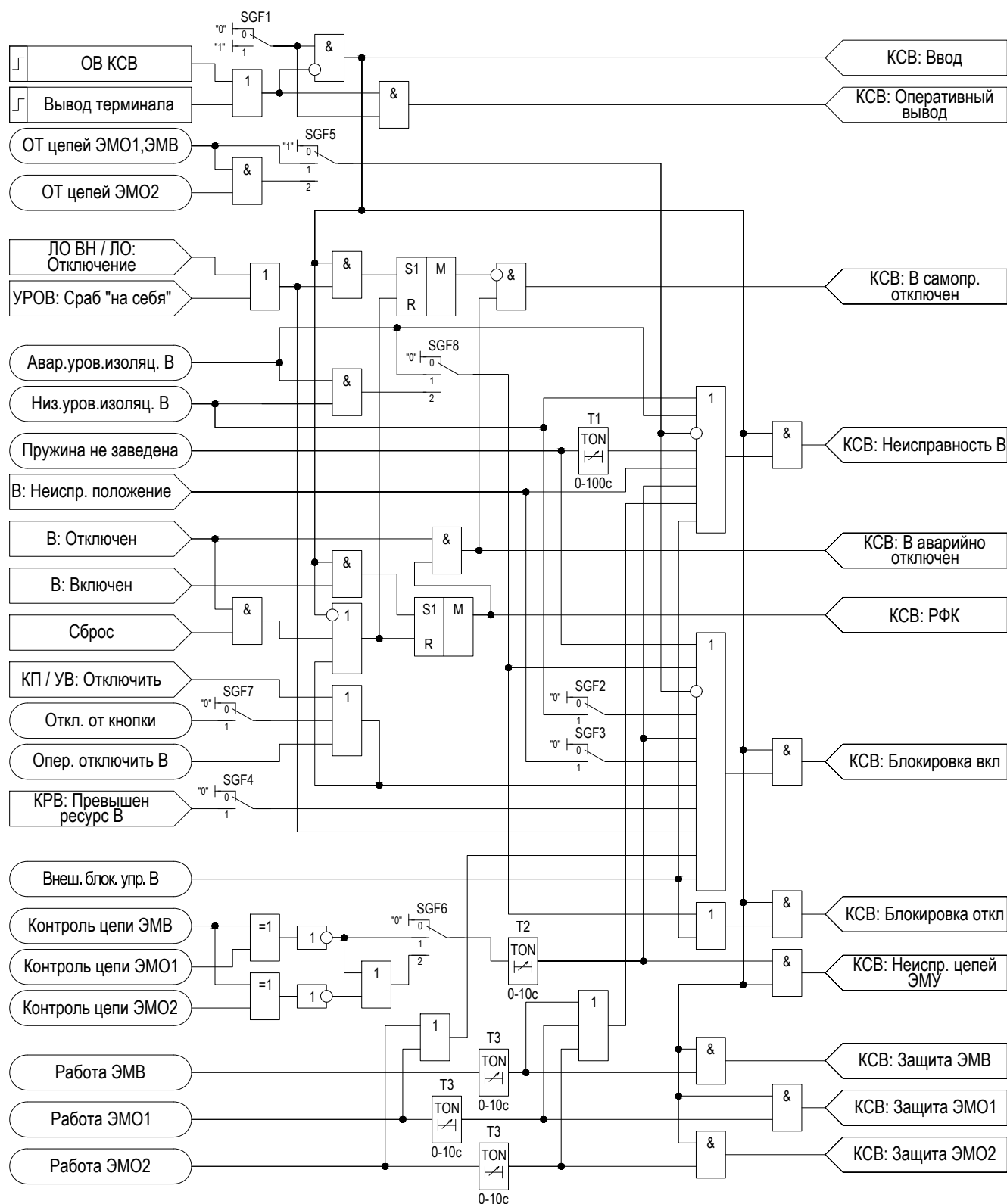
Рисунок 2.22 – Функциональная схема логики КСВ
