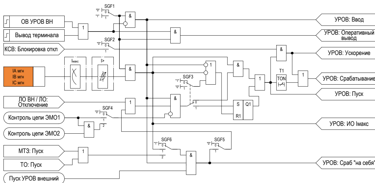
Рисунок 2.20 – Функциональная схема логики УРОВ
