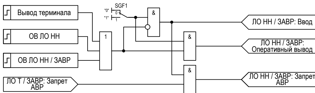
Рисунок 2.19 – Функциональная схема логики запрета АВР
