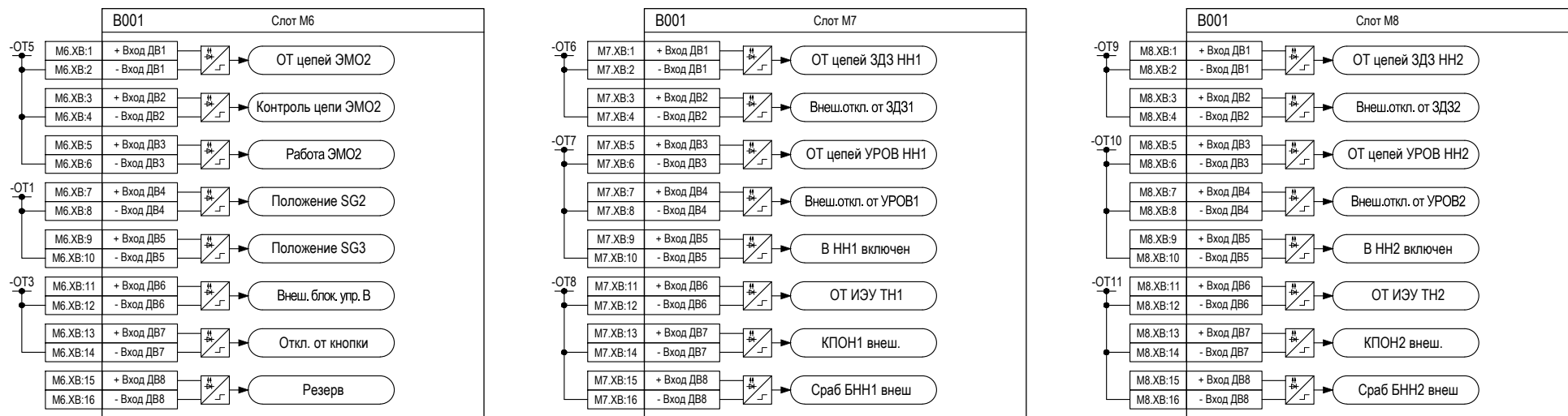
Рисунок Г.3 – Подключение дискретных входов и выходов к внутренним сигналам алгоритмов для блоков в слотах М6-М8
