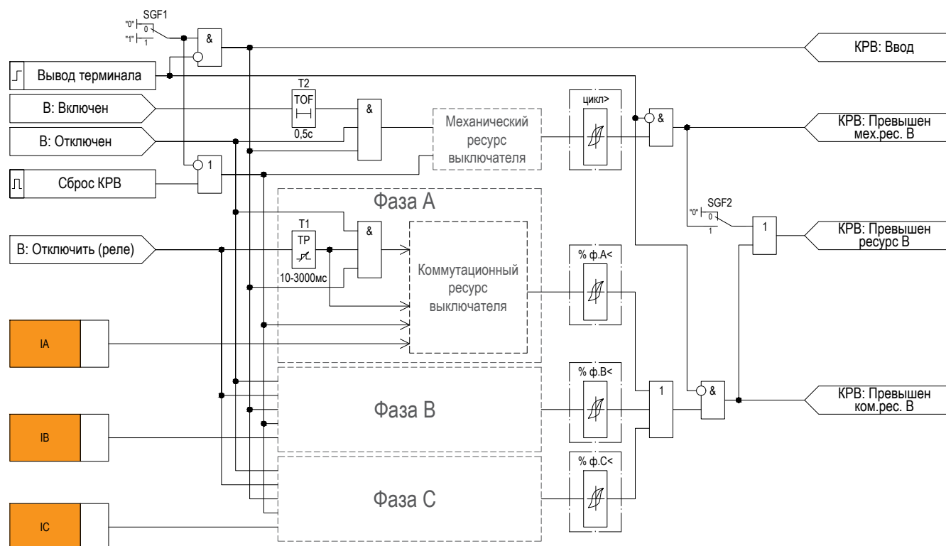
Рисунок 2.21 – Функциональная схема логики КРВ
