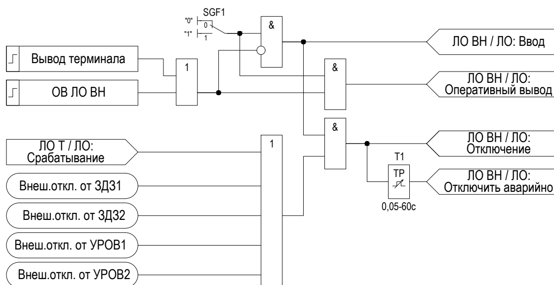
Рисунок 2.16 – Функциональная схема ЛО ВН
