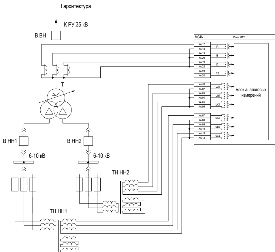
Рисунок В.2 – Подключение аналоговых цепей трансформаторов тока и напряжения трансформатора 35 кВ с расщепленной обмоткой низшего напряжения к устройству
